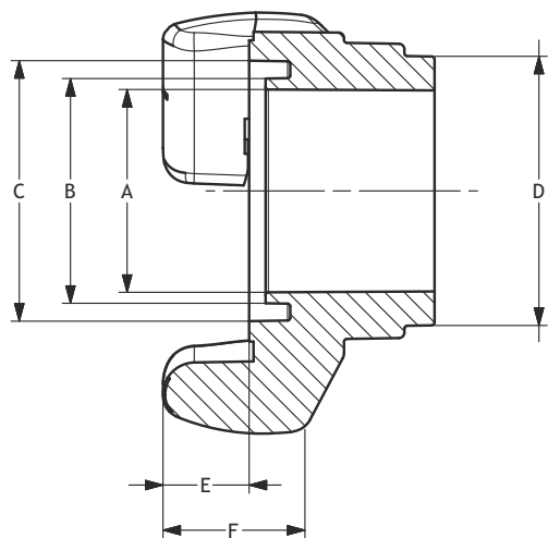
SECCION A-A
