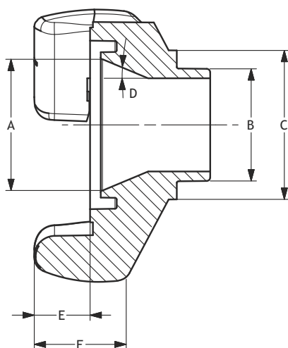
SECCION A-A
